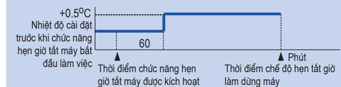
Nhiệt độ phòng gia tăng lên 0,5°C sau 60 phút, nhưng vẫn duy trì mức độ ổn định nhất ở dàn nóng.
